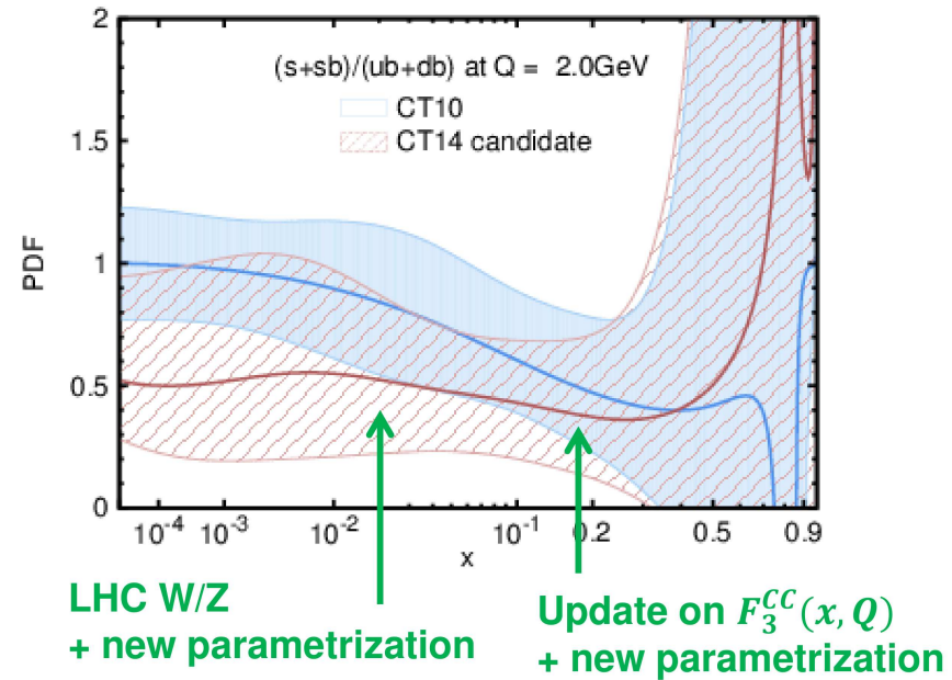
CTx PDF SET
